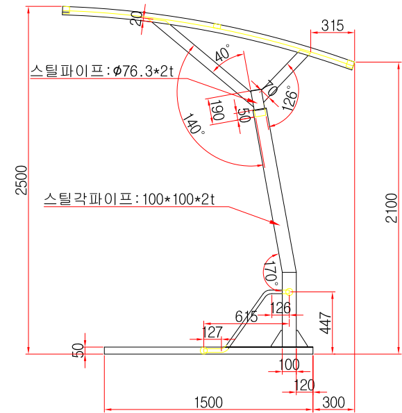
⊕ SIDE ELEVATION SCALE: NONE
